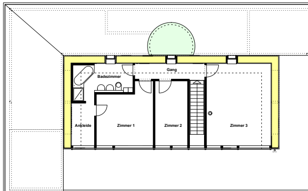
Grundriss Obergeschoss
