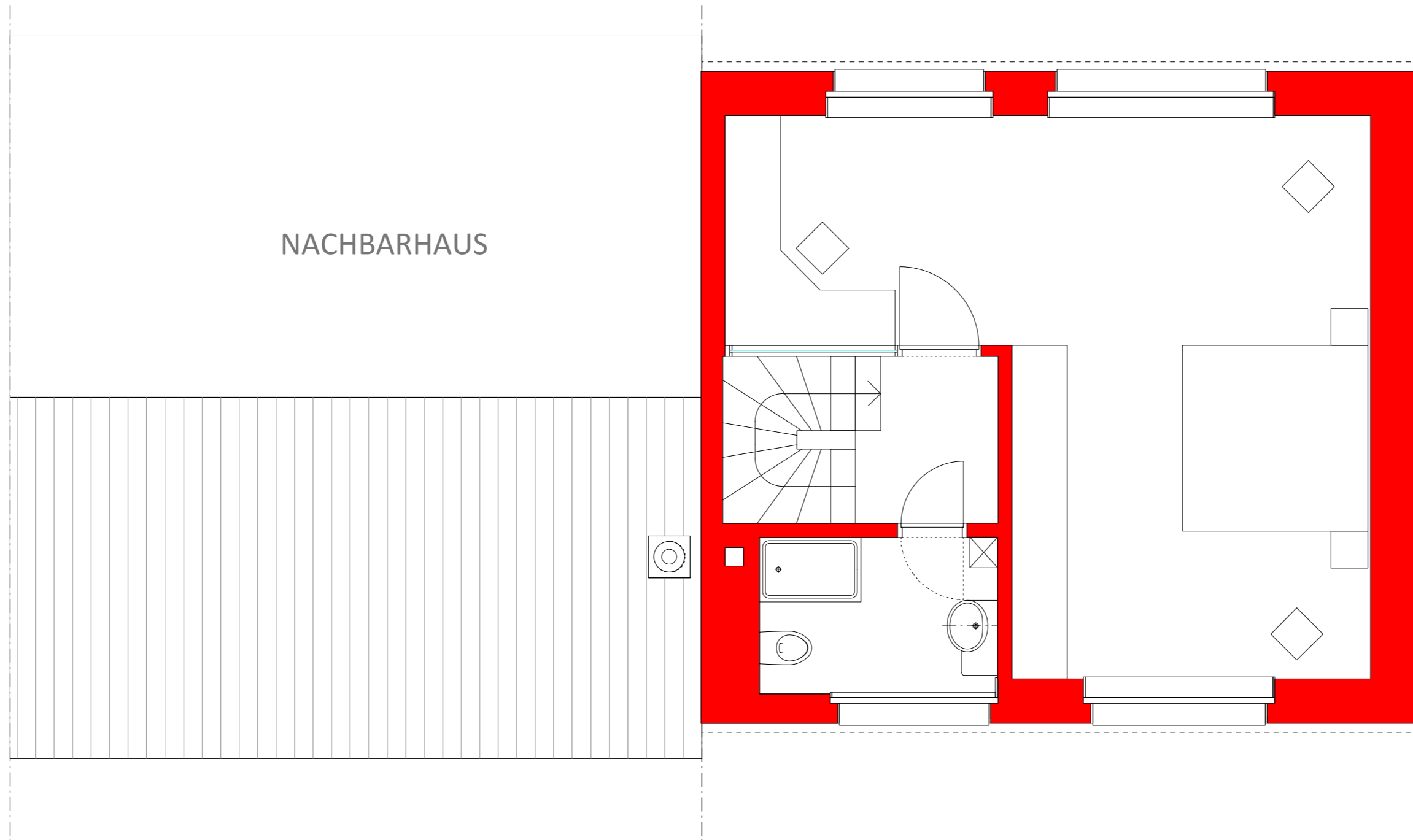
GRUNDRISS DACHGESCHOSS
