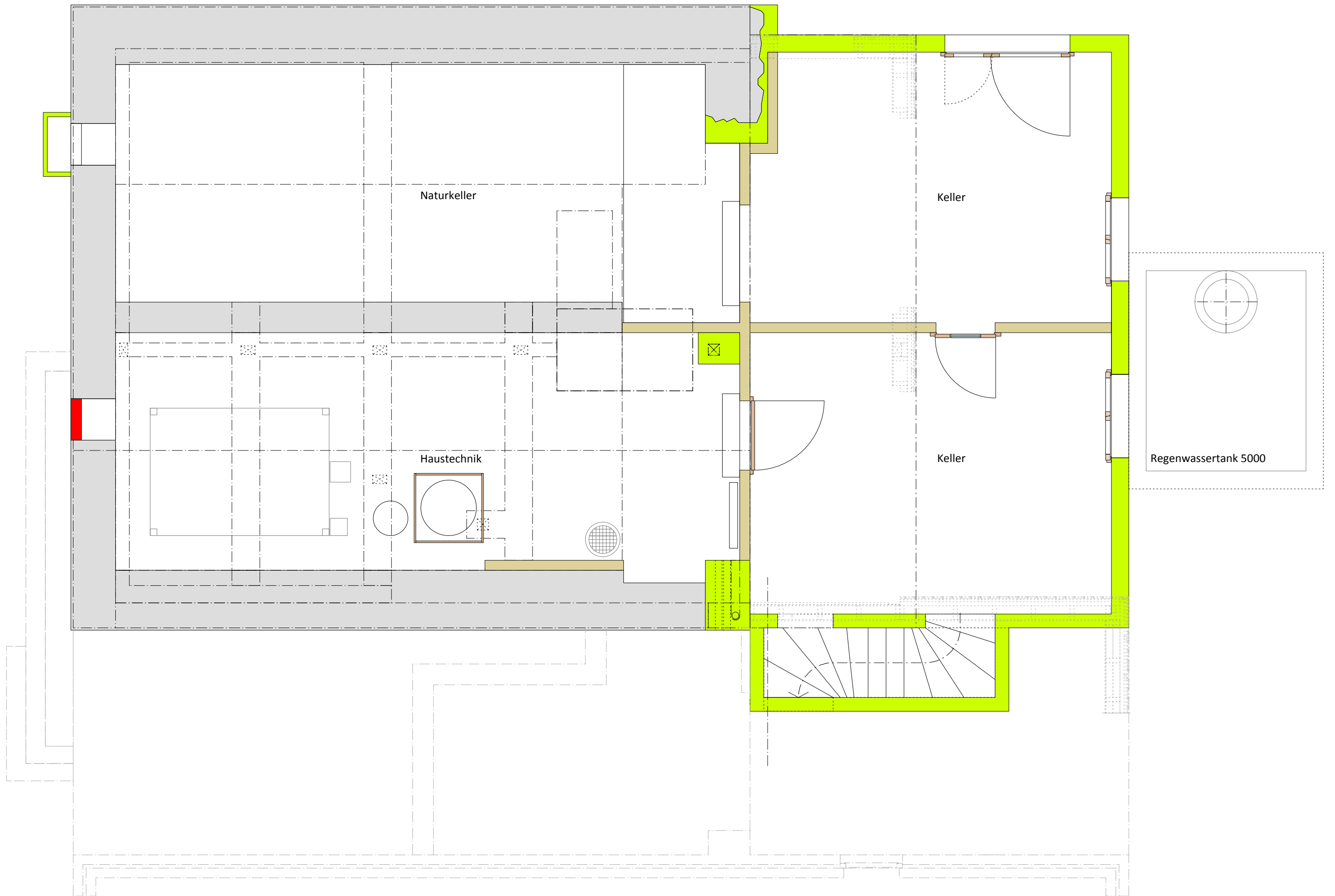
Kellergeschoss
