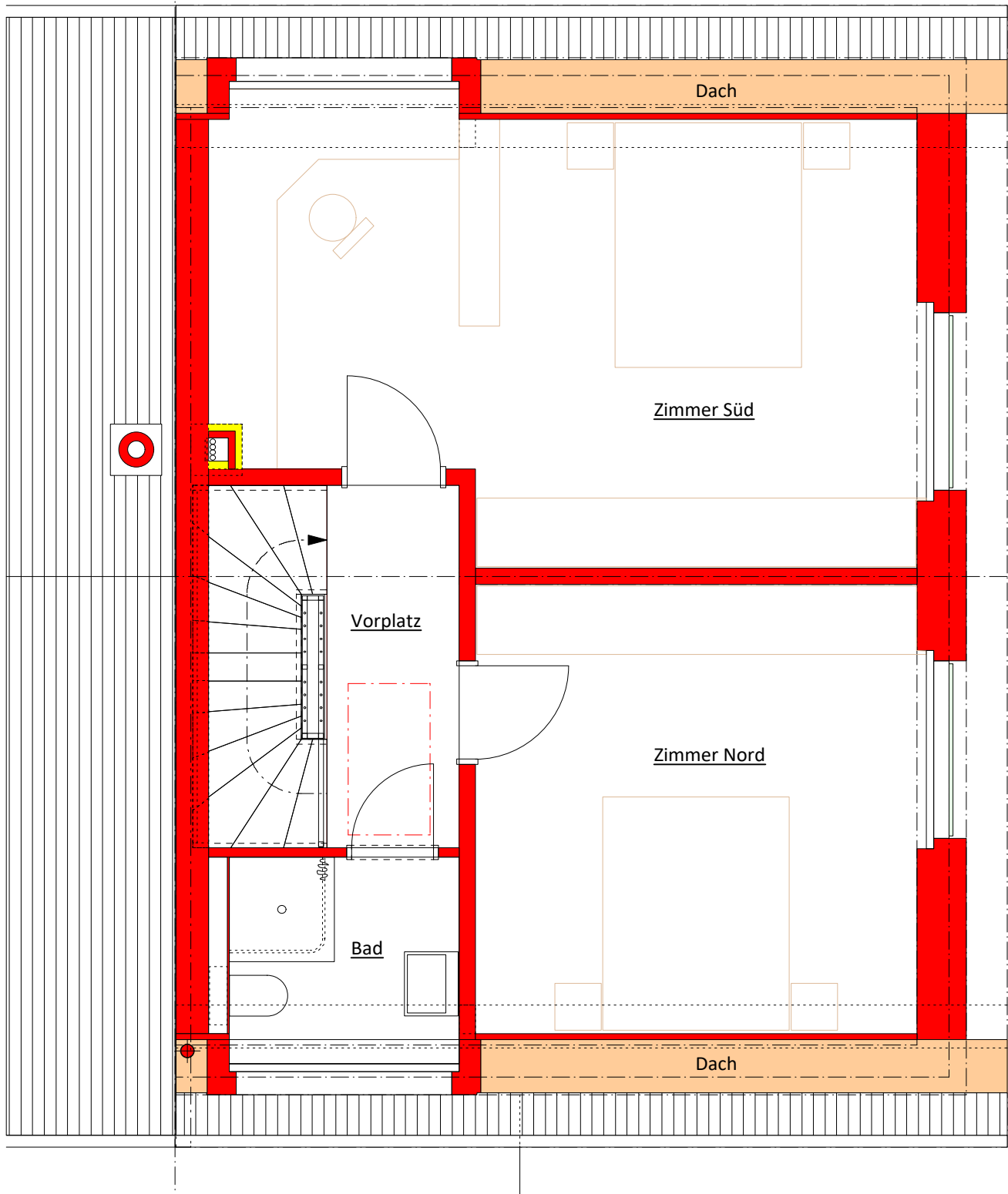
Grundriss Dachgeschoss NEU
